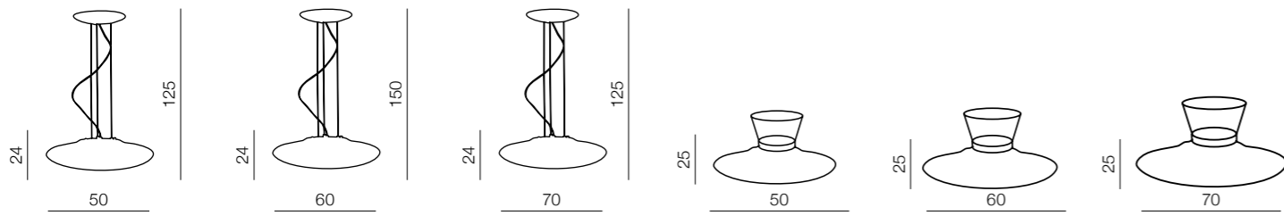
Pires 50 AZ0277 E27 3x 60W metal/glass chrome/white Pires 60 AZ0278 E27 4x 60W metal/glass chrome/white Pires 70 AZ0279 E27 5x 60W metal/glass chrome/white Pires 50 top AZ0280 E27 3x 60W metal/glass chrome/white Pires 60 top AZ0281 E27 4x 60W metal/glass chrome/white Pires 70 top AZ0282 E27 5x 60W metal/glass chrome/white
