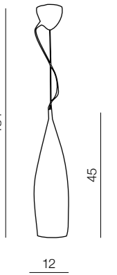
Testa AZ0120 E27 1x 40W metal/glass chrome/white
