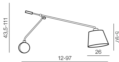
Sevilla LAMP BODY + ZF OR DS SHADES 1x E27 MAX 60W metal/fabric
